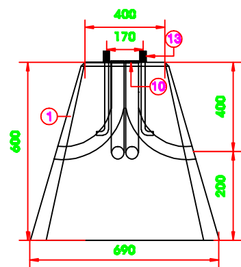
정면도
