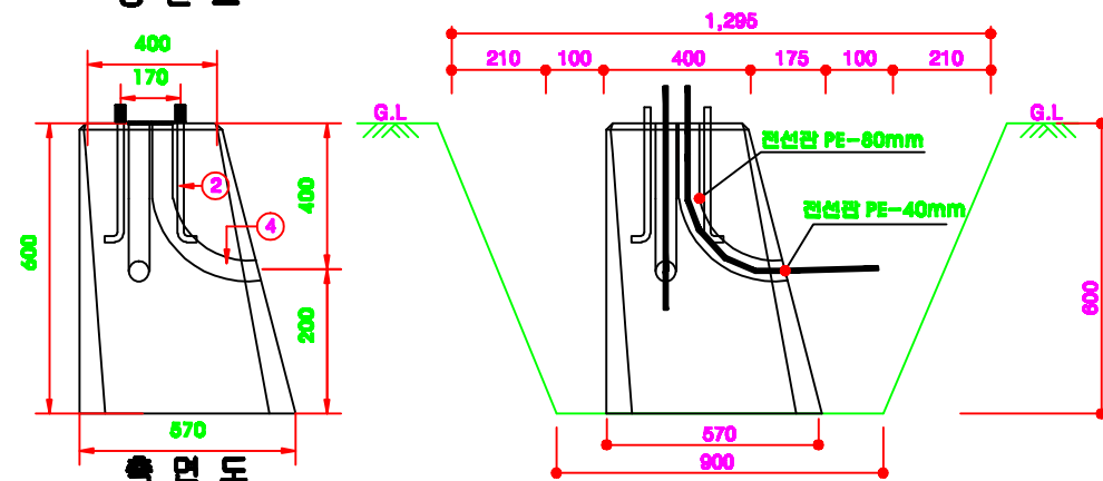
측면도
