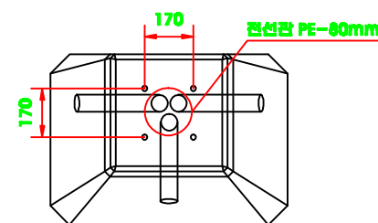
주책기반 / 보안등 기초 상세도
