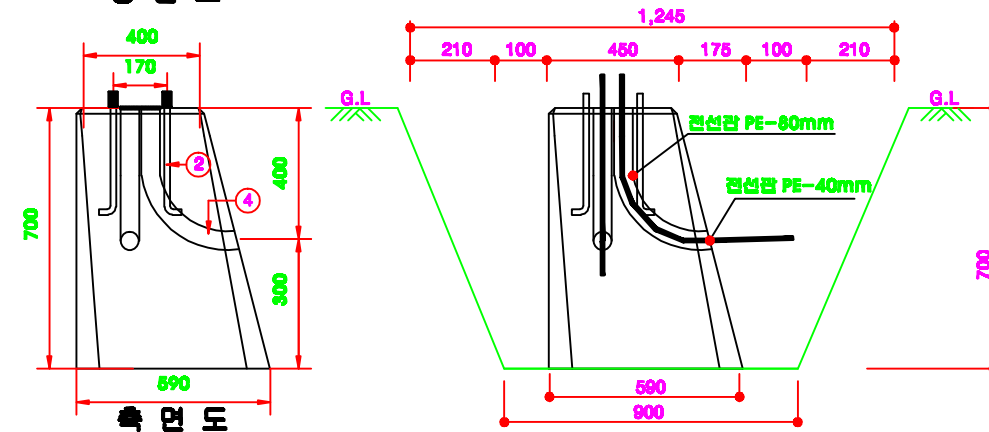
주책기반 / 보안등 기초 상세도
