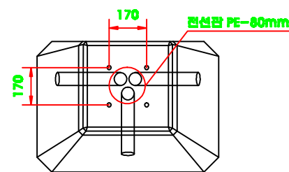
평면도
