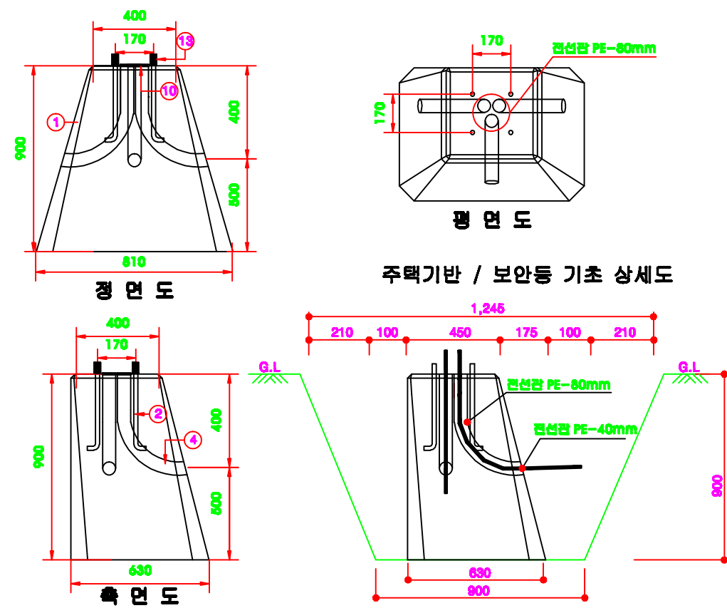
면처리기초상세도 (400x810x630x900)
