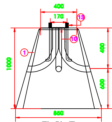
정면도
