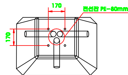
평면도
