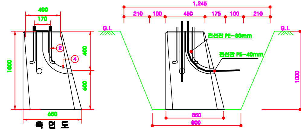
측면도
